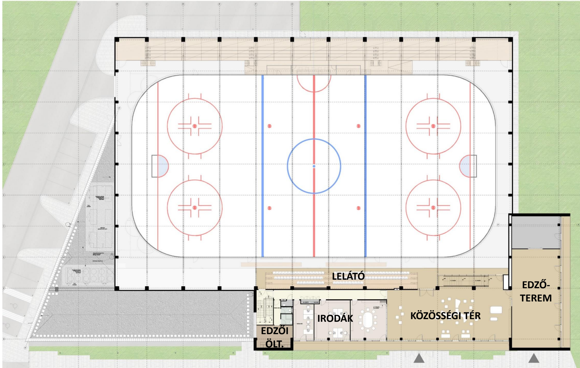
EMELETI ALAPRAJZ
