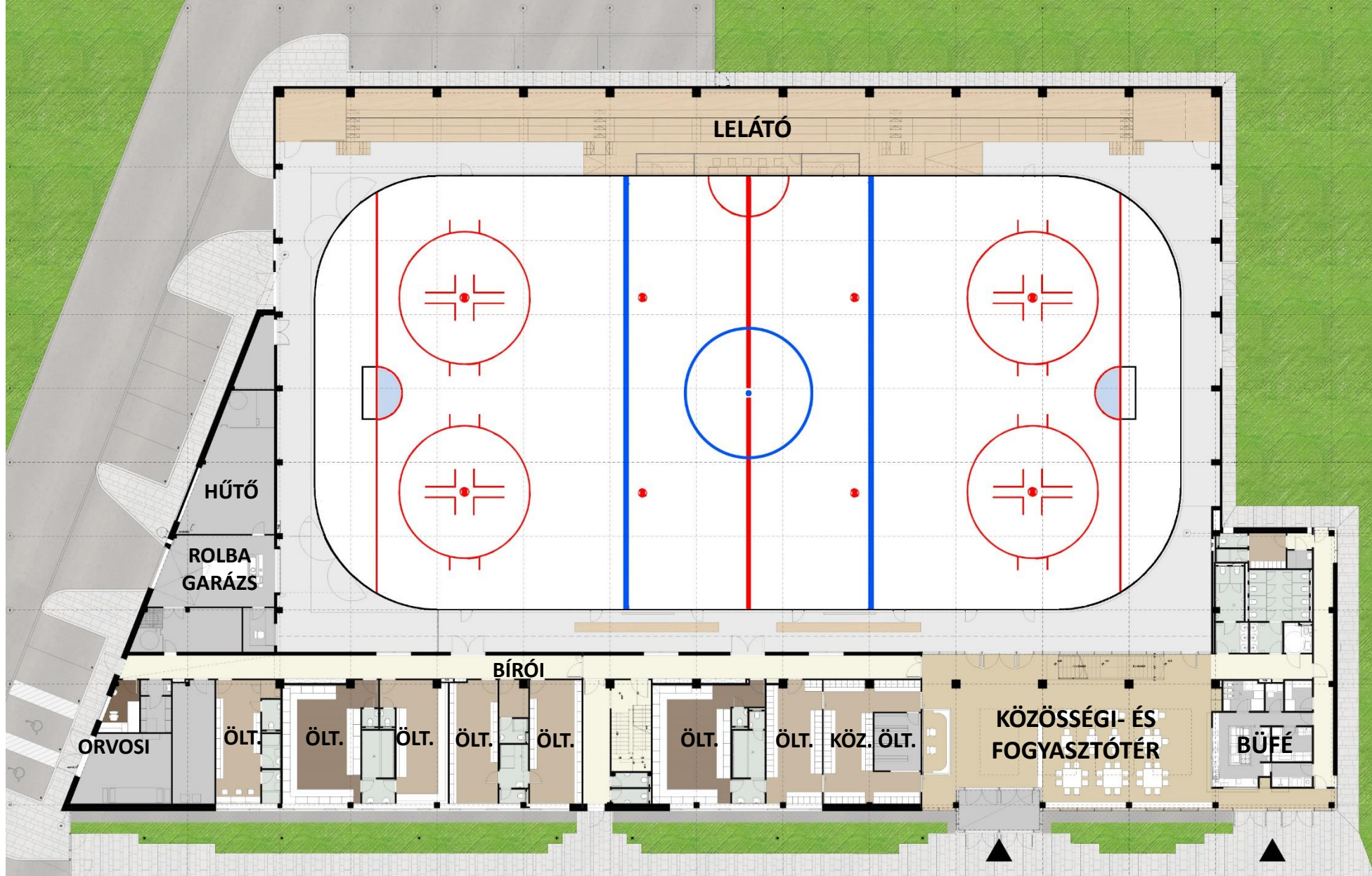
FÖLDSZINTI ALAPRAJZ
